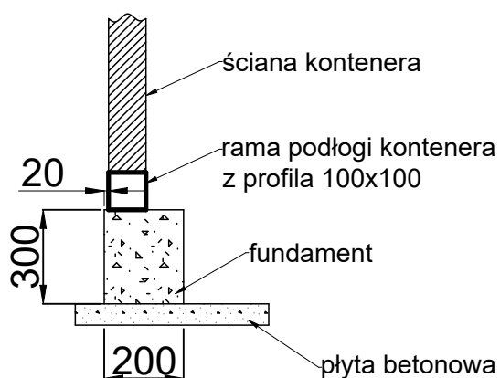
segment nr 1 na fundamencie
