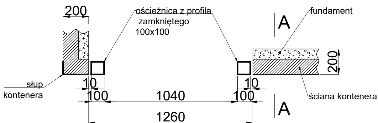
szczegół A segm nr 1
